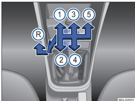
图 111 5 挡手动变速箱挡位示意图
