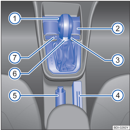
图 7 中控台下部分概览
