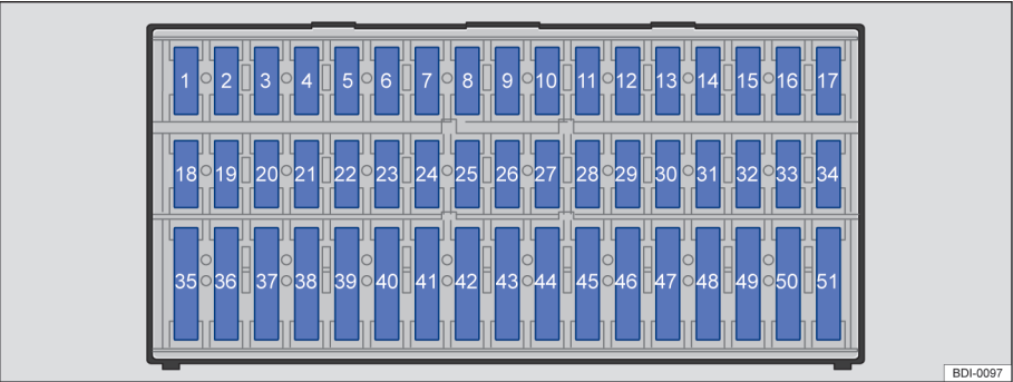
图 167 保险丝盒中的保险丝
