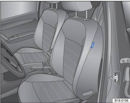
图 70 前座椅上侧面：侧面安全气囊的安装位置
