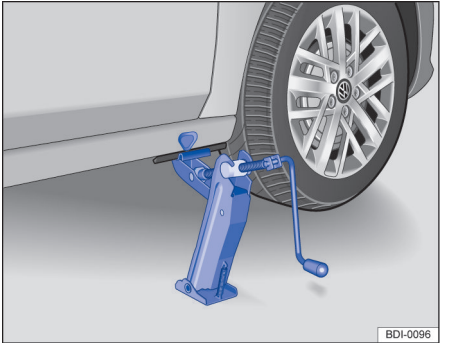
图 164 将千斤顶放在汽车左后侧
