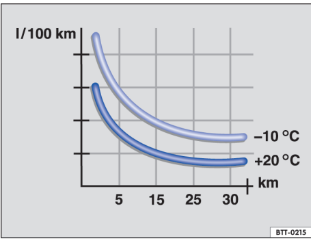
图 114 两种不同环境温度时的百公里油耗
