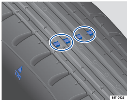
图 144 轮胎花纹磨损标记
