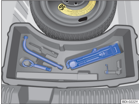
图 155 部分车型行李厢盖板下部的随车工具
