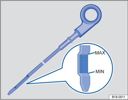
图 138 带液位标记的机油标尺
