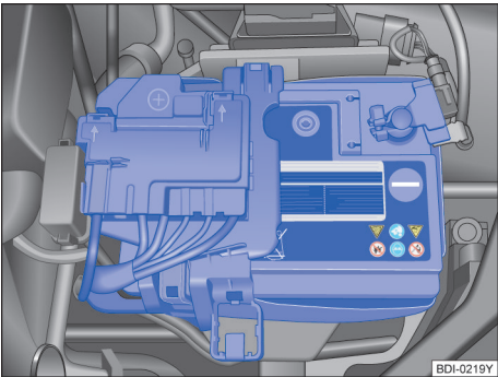
图 141 蓄电池
