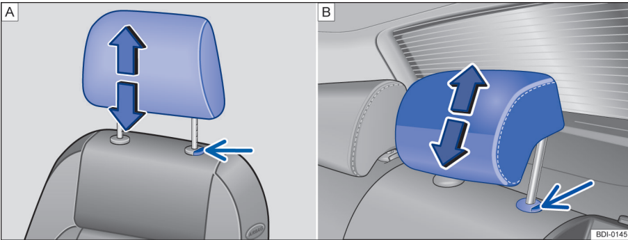
图 51 A 前排头枕拆卸和安装、B 调整后排头枕
