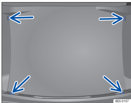
图 91 行李厢局部视图：固定环
