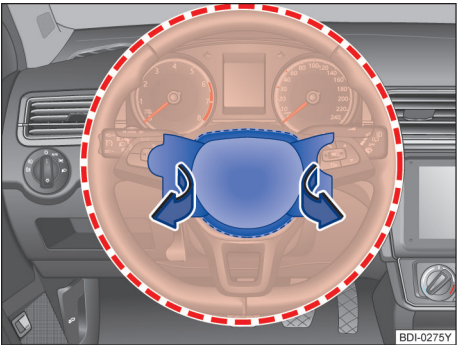
图 68 前排正面安全气囊的安装位置和膨胀范围
